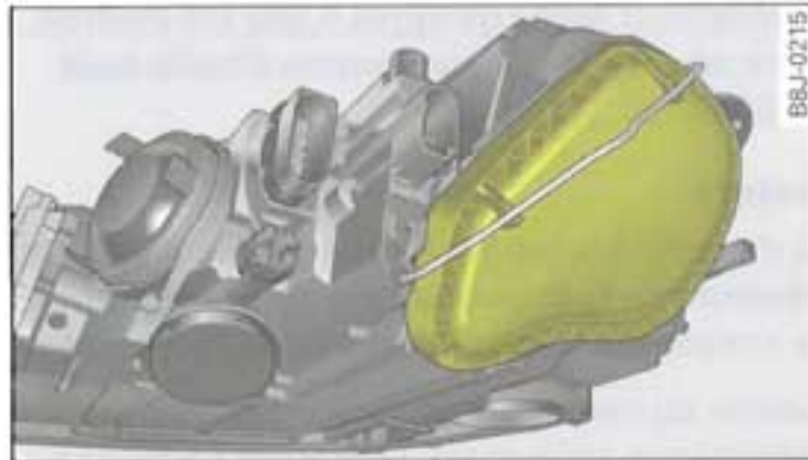
Fig. 141 Phares halogènes avec cache fermé
