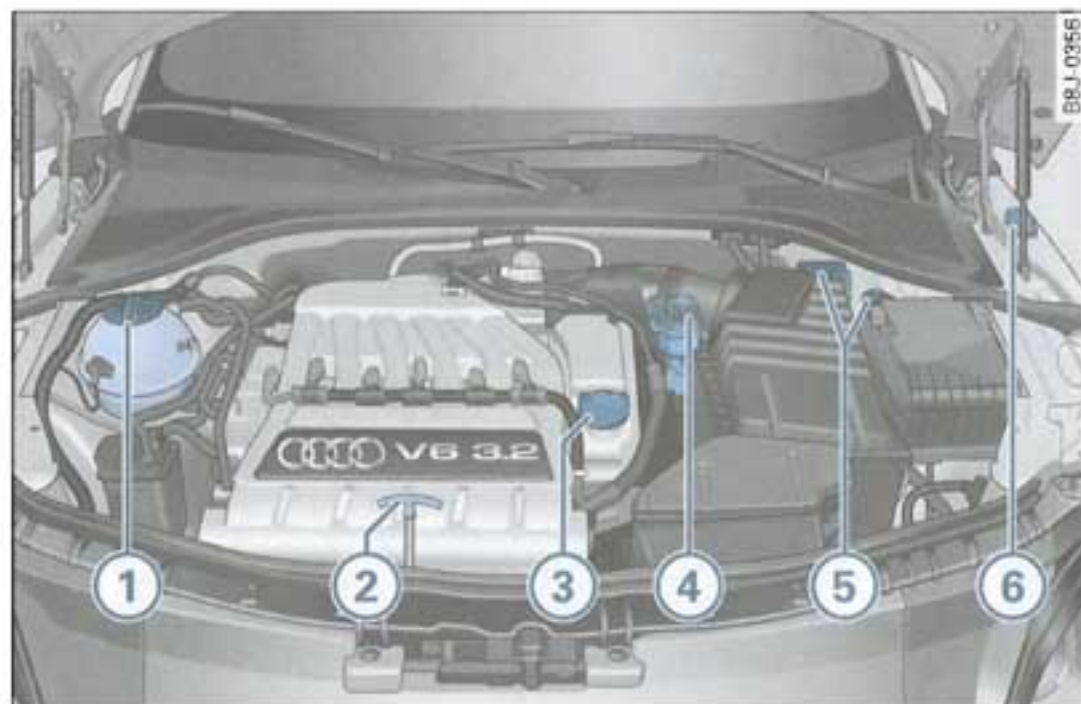
Fig. 149 Agencement des réservoirs, de la jauge d'huile-moteur et de l'ajutage de remplissage d'huile-moteur
