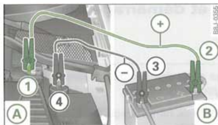
Fig. 175 Aide au démarrage avec la batterie d'un autre véhicule : A : batterie déchargée, B : batterie fournissant le courant
