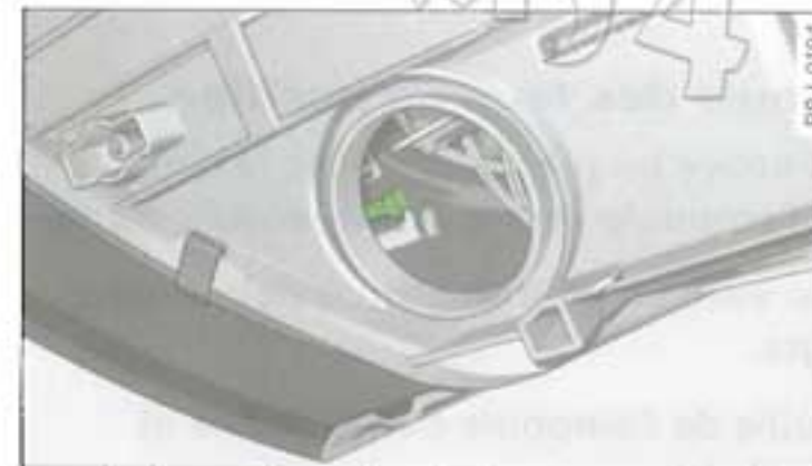
Fig. 188 Capuchon en caoutchouc ouvert : accès au feux de position
