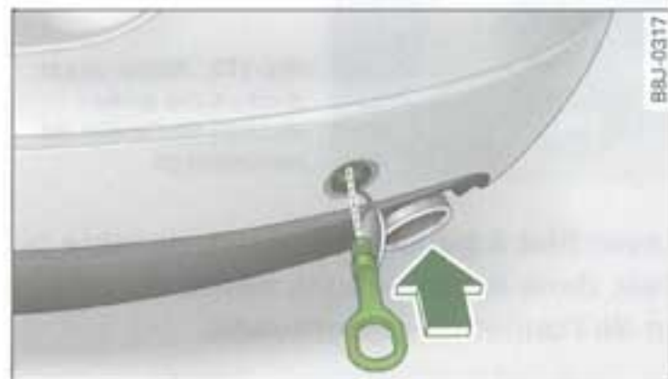
Fig. 178 Partie arrière droite : vissage de l'œillet de remorquage
