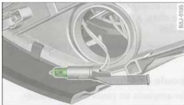
Fig. 189 Retirez la douille de l'ampoule (feux de position)
