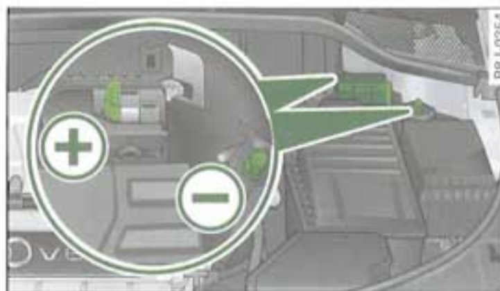
Fig. 174 Vous disposez d'un dispositif d'aide au démarrage dans le compartiment-moteur, côté gauche, pour l'aide au démarrage et pour la recharge de la batterie.
