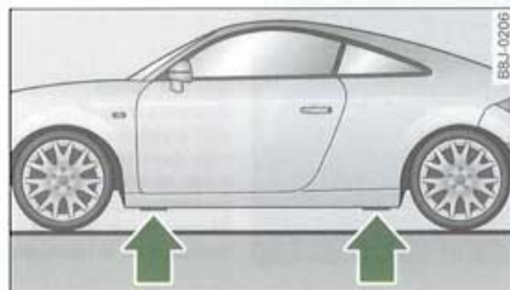
Fig. 172 Changement de roue : points d'appui du cric
