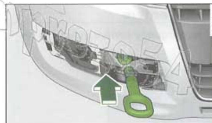
Fig. 177 Partie avant droite sans grille : vissage de l'œillet de remorquage
