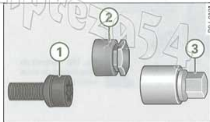
Fig. 171 Boulon de roue antivol avec capuchon de protection et adaptateur
