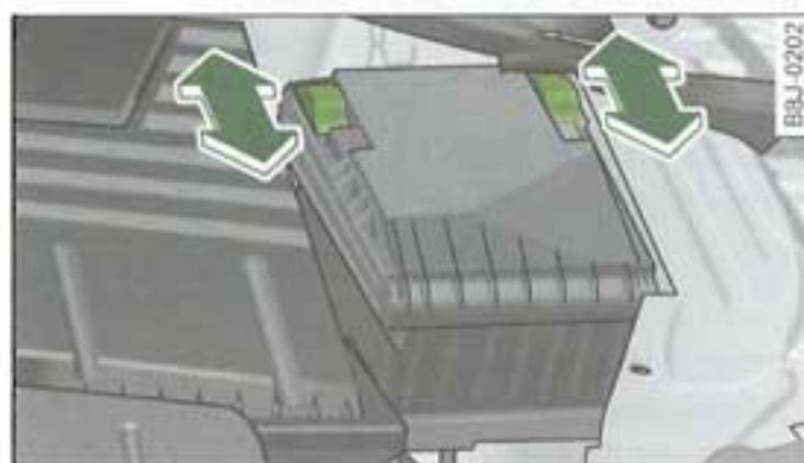
Fig. 180 Compartiment-moteur, côté gauche : couvercle des fusibles
