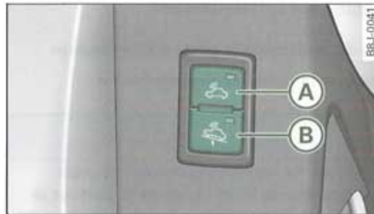
Fig. 45 Commande du dispositif de surveillance de l'habitacle dans le revêtement de la porte (uniquement visible lorsque la porte du conducteur est ouverte).
