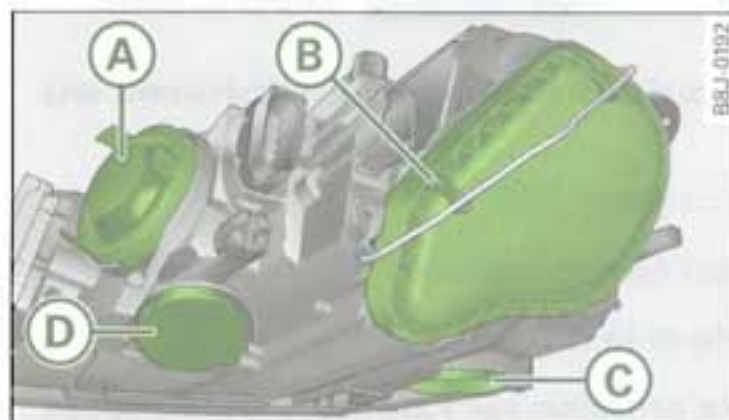
Fig. 183 Emplacement des ampoules dans le phare droit
