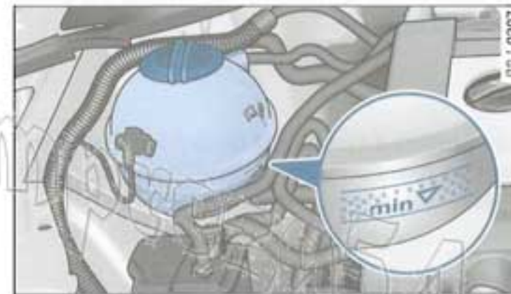
Fig. 153 Compartiment-moteur : repères sur le vase d'expansion de liquide de refroidissement
