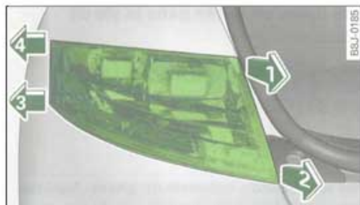
Fig. 194 Dépose du feu arrière
