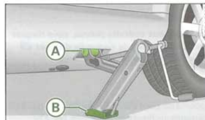
Fig. 173 Changement de roue : cric
