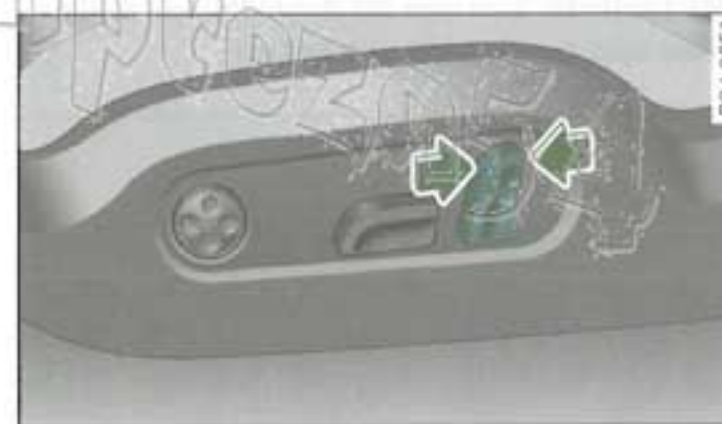
Fig. 71 Siège avant : commande d'inclinaison du dossier
