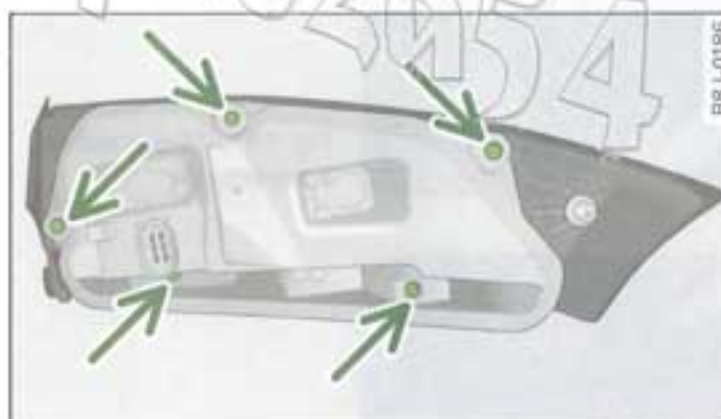
Fig. 195 Feu arrière avec support d'ampoules
