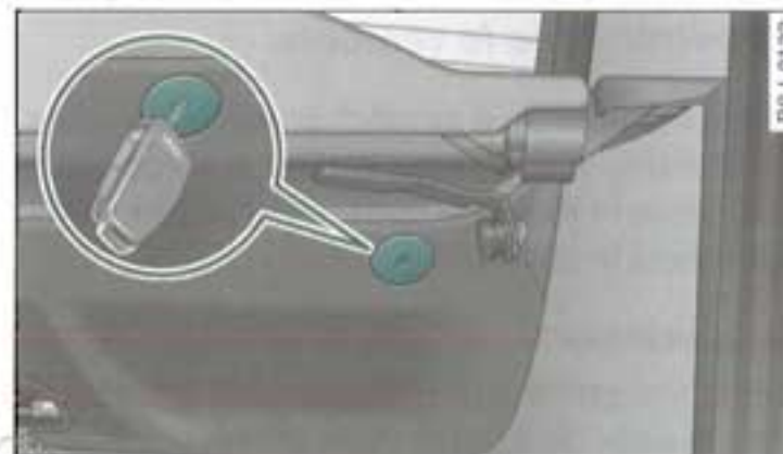
Fig. 43 L'accès au déverrouillage d'urgence se situe sous la lunette arrière, à gauche dans le coffre à bagages.
