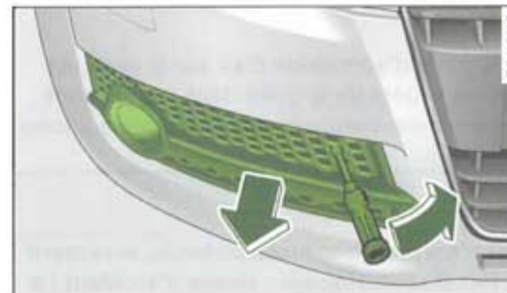
Fig. 176 Partie avant droite : démontage de la grille d'admission d'air
