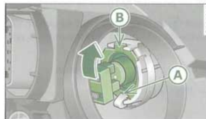
Fig. 185 Boîtier de l'ampoule : mise en place de l'ampoule
