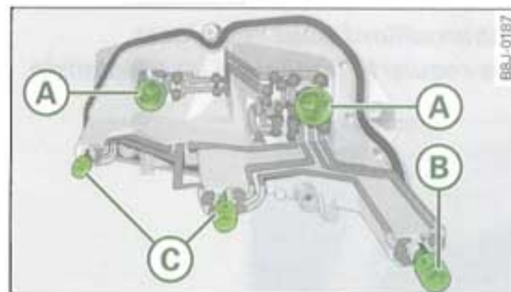
Fig. 196 Emplacement des ampoules sur le support d'ampoules. Exemple : feu arrière gauche
