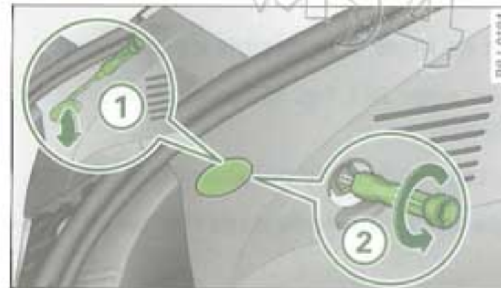
Fig. 193 Coffre à bagages : vis de fixation de feu arrière
