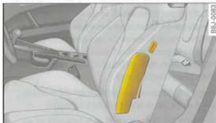
Fig. 126 Emplacement de montage de l'airbag latéral dans le siège conducteur
