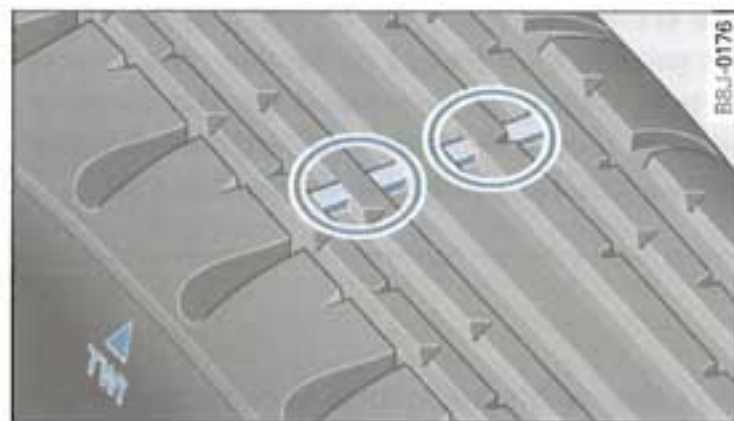
Fig. 159 Sculptures de pneu : Indicateurs d'usure
